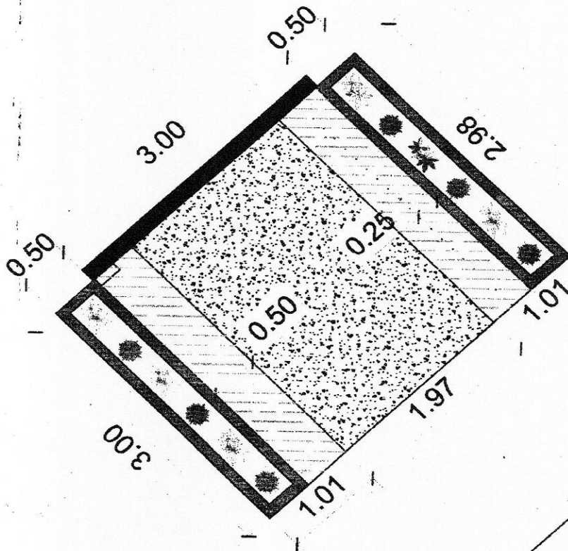
PLANTA
