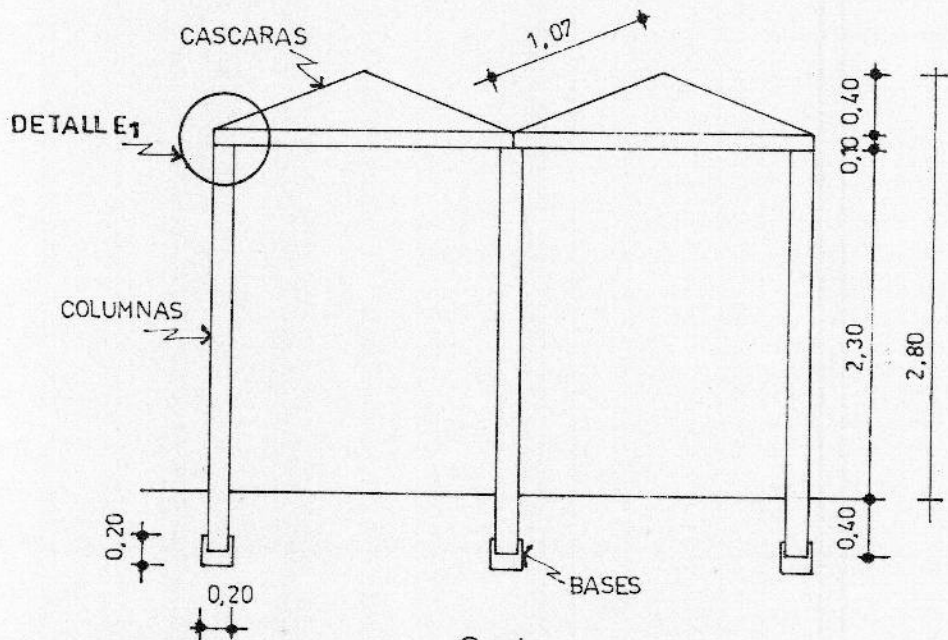
Corte Esc 1:50
