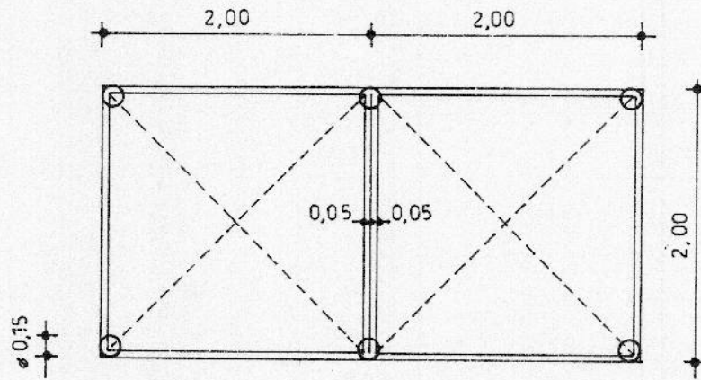
Planta Esc 1:50
